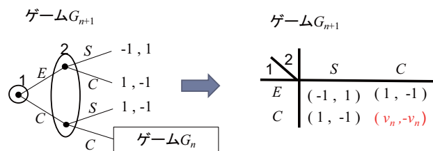
図 5.7: ゲーム G_{n+1}
