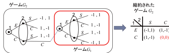
図 5.6: ゲーム G_2
