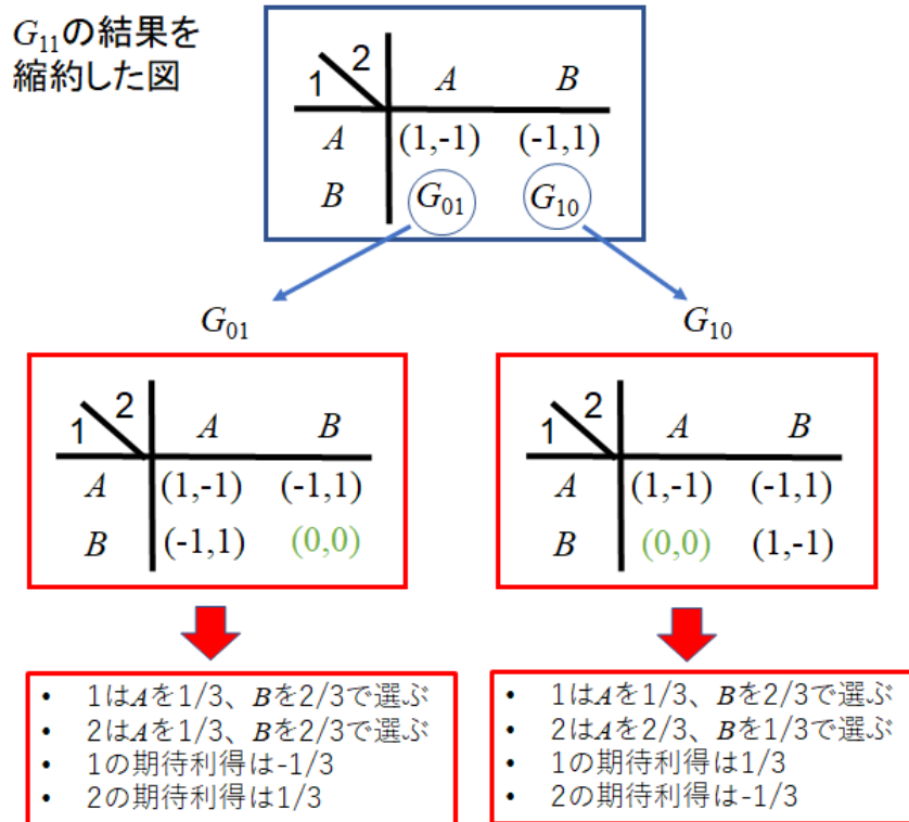
図 5.3: G_{11} を縮約し G_{01} と G_{10} を解いた図
